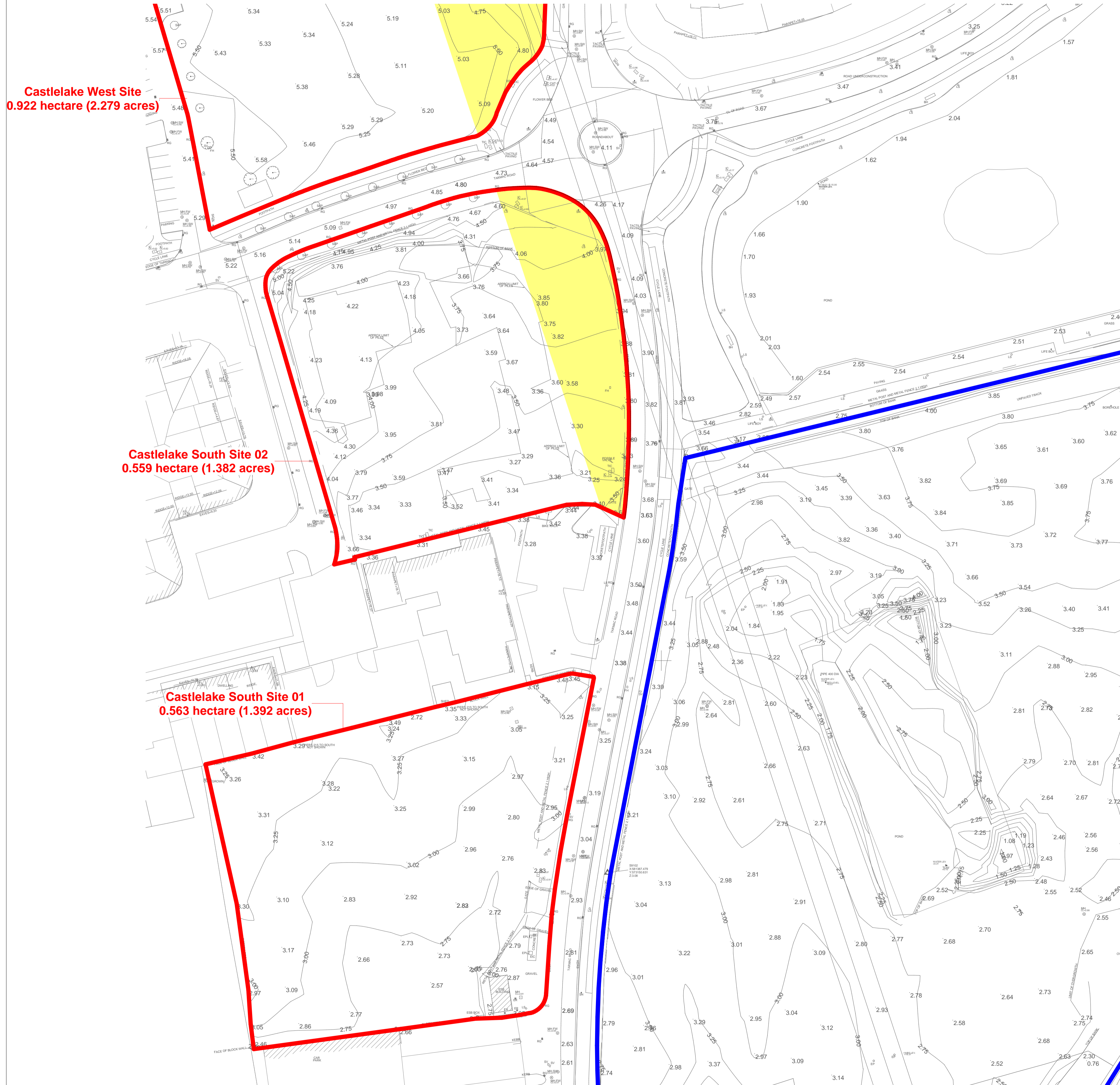
1 Existing Site Survey 01 1 : 500
